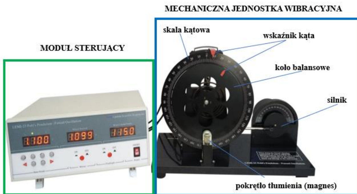
Rys. 1. Opis aparatury pomiarowej.
