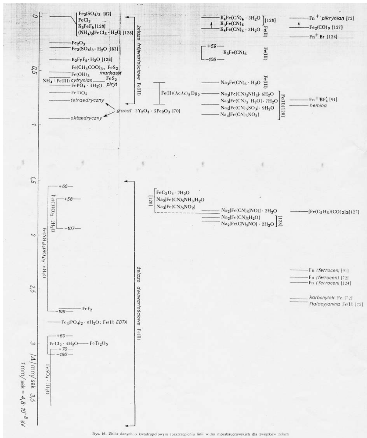
Rys. 16. Zbiór danych o kwadrupolowym rozszczepieniu linii widni móssbauerowskich dla związków żelaza
